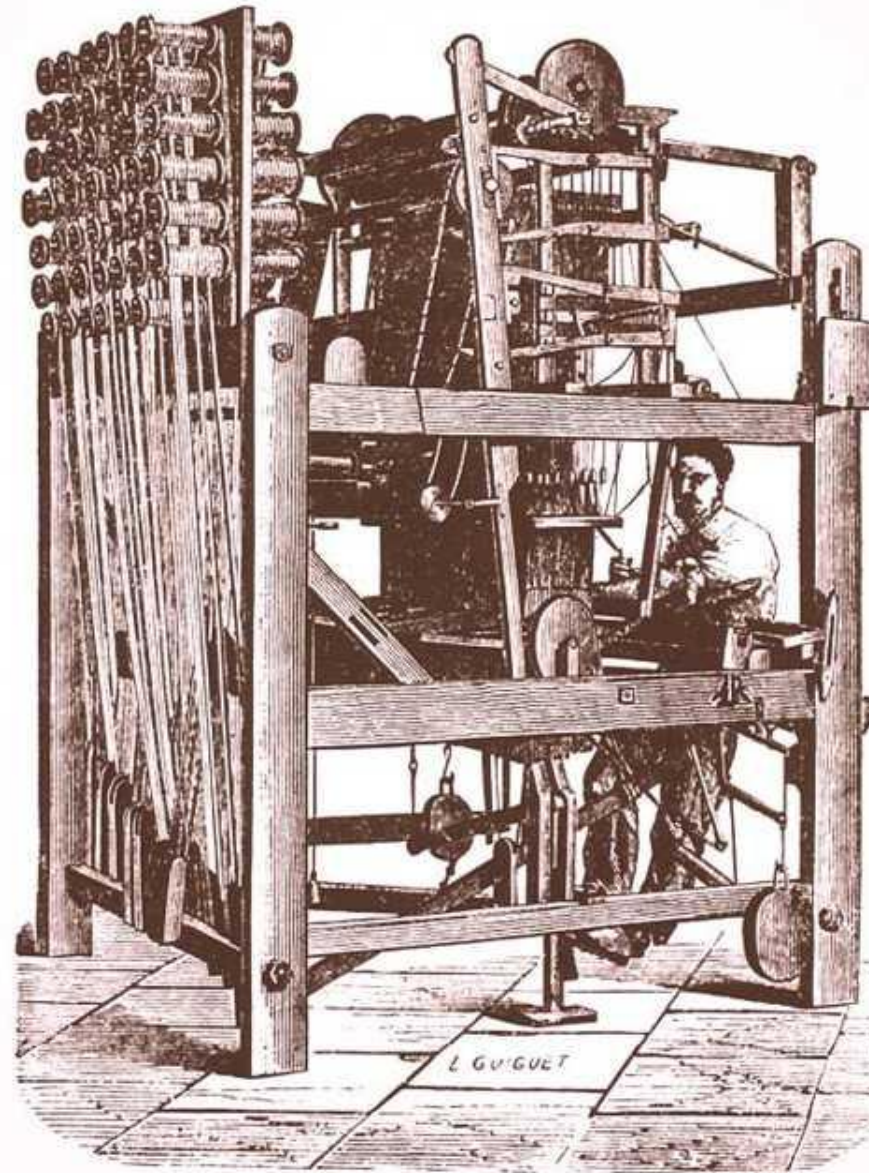
MÉTIER DE JEAN WERLY PERFECTIONNÉ, POUR LA FABRICATION MÉCANIQUE DES CORSETS SANS COUTURES, AYANT APPARTENU A L'ANCIENNE MAISON LIBRON ET STIEGLER, BAR-LE-DUC, 1875.
